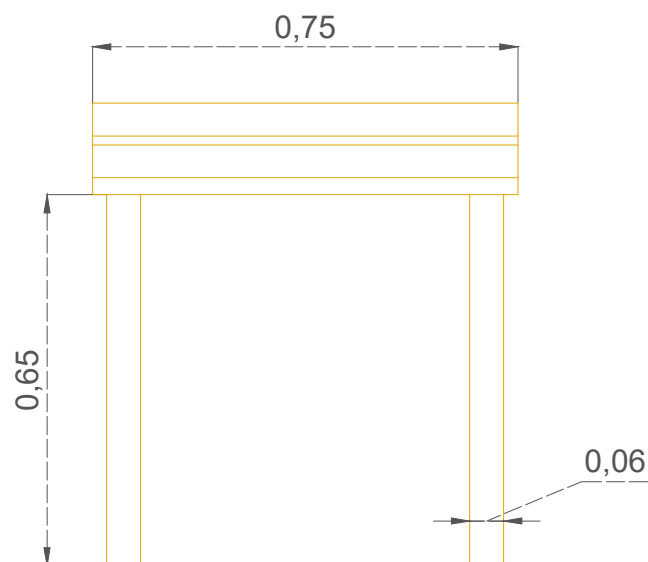
Alzado
