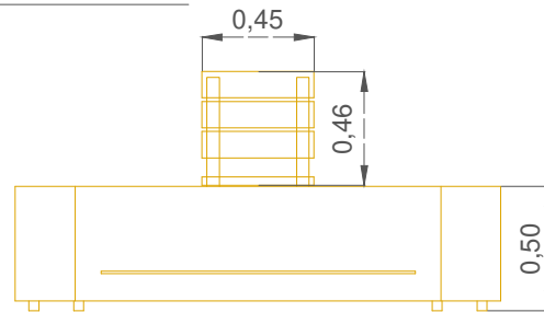
Alzado frontal
